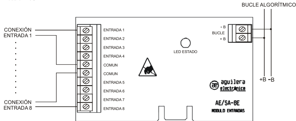
Módulo AE/SA-8E
