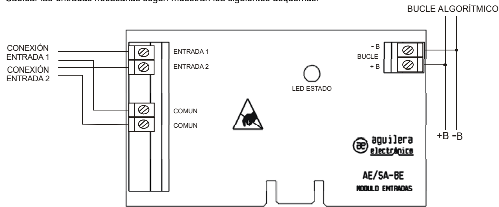
Módulo AE/SA-2E
